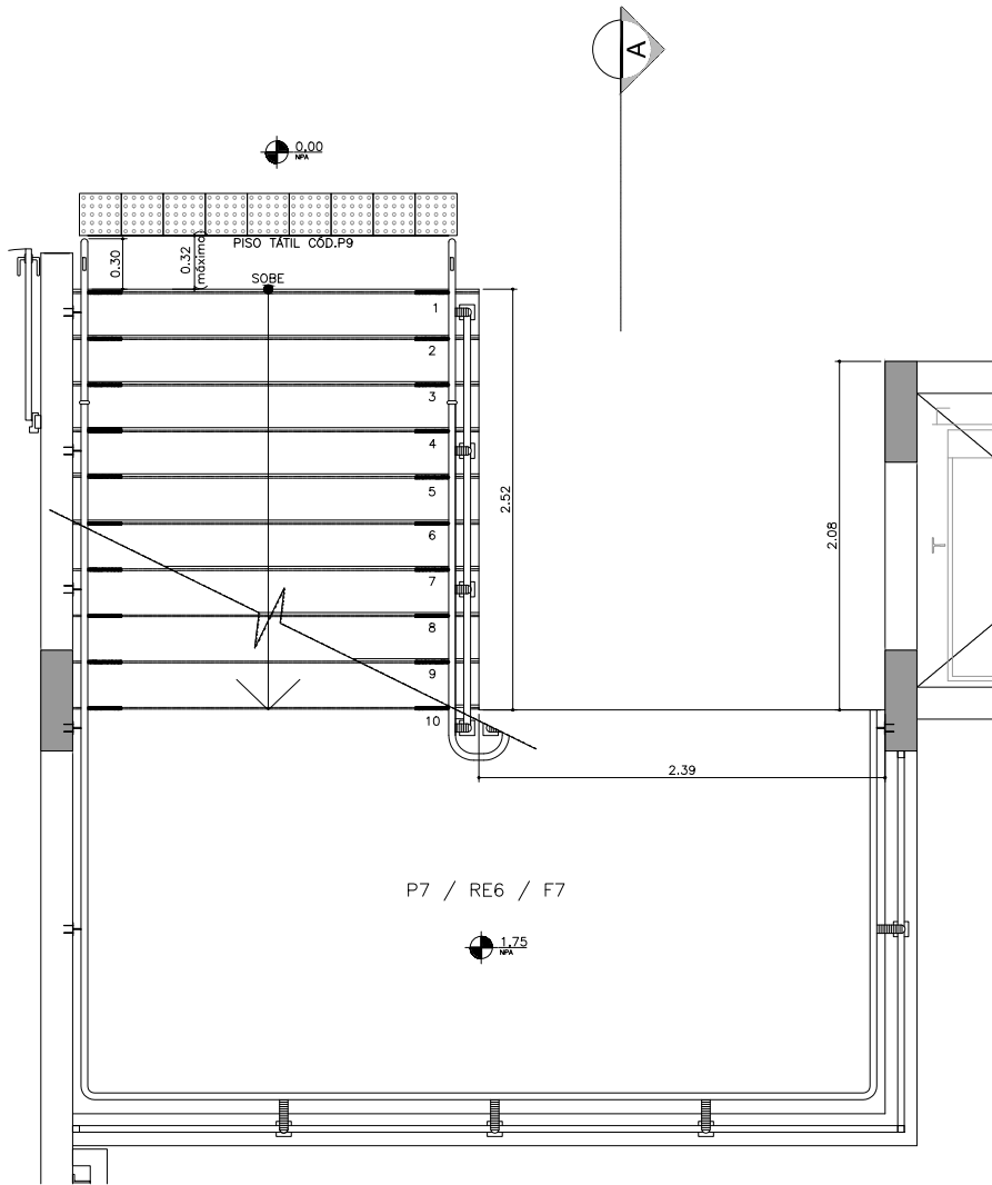
1 ESCADA - SALA DE AULAS Planta Nível 0,00 ESCALA: SEM ESCALA
