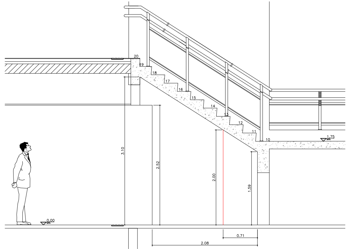
2 ESCADA Corte A ESCALA: SEM ESCALA
